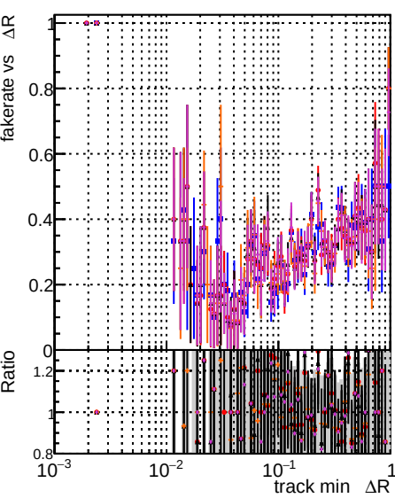
Fake rate vs \Delta R(\text{track, jet}) Legend: DOM CKFit 1000evt DOM CKFit 10000evt DOM CKFit 100000evt DOM CKFit 1000000evt TEST OHIT 10000evt TEST OHIT 100000evt TEST OHIT 500000evt
