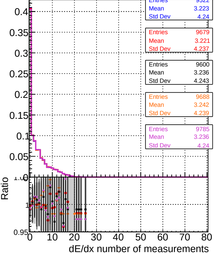
DOM CKFFit 1000evt DOM CKFREFit 1000evt DOM MkFitREFit 1000evt DOM TESTOLHIT 1000evt DOM TESTOLHIT 1000evt-50000t
