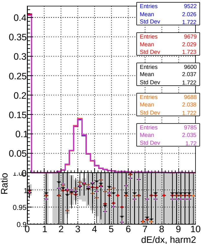
DOM CKFFit 1000evt DOM CKFREFit 1000evt DOM MkFitREFit 1000evt DOM TESTOLHIT 1000evt DOM TESTOLHIT 1000evt-50000t
