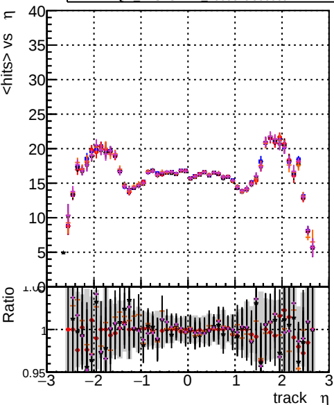
mean hits vs \eta DOM CKFEEIT 1000evt DOM CKFEEIT 1000evt DOM CKFEEIT 1000evt DOM TESTOLHIT 1000evt DOM TESTOLHIT 1000evt-50000t
