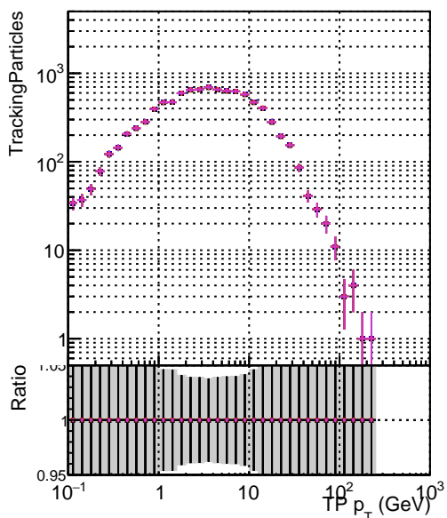
— DQM CKEEFIT 1000evt — DQM CKEEFIT 10000evt — DQM CKEEFIT 100000evt — DQM TESTOLHIT 1000evt — DQM TESTOLHIT 10000evt — DQM TESTOLHIT 100000evt
