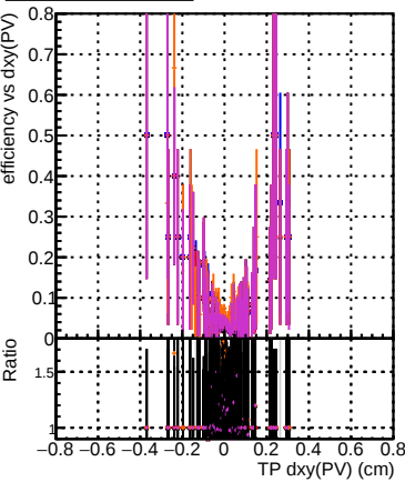
Efficiency vs Dxy(PV) DQM_CKFFit_1000evt DQM_CKFREFit_1000evt DQM_MkFitREFit_1000evt DQM_TESTOLHIT_1000evt DQM_TESTOLHIT_1000evt-50000t
