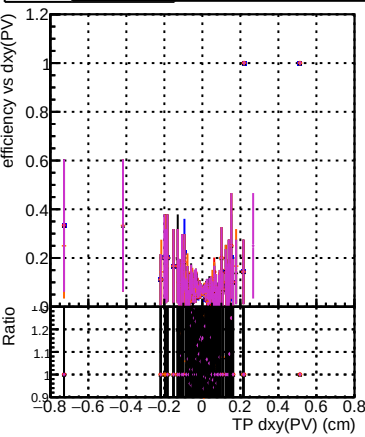
Efficiency vs Dxy(PV) (cm) Legend: DQM_CKFit_1000evt DQM_CKFREFit_1000evt DQM_MkFitREFit_1000evt DQM_TESTOLHIT_1000evt DQM_TESTOLHIT_1000evt-50000t
