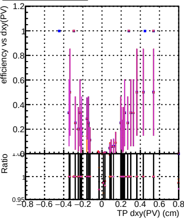
Efficiency vs Dxy(PV) Legend: DOM_CKFFit_1000evt DOM_CKFREFit_1000evt DOM_MkFitREFit_1000evt DOM_TESTOLHIT_1000evt DOM_TESTOLHIT_1000evt-50000t
