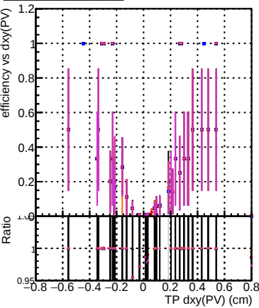
Efficiency vs Dxy(PV) Legend: DQM_CKFFit_1000evt DQM_CKFREFit_1000evt DQM_MkFitREFit_1000evt DQM_TESTOLHIT_1000evt DQM_TESTOLHIT_1000evt-50000t
