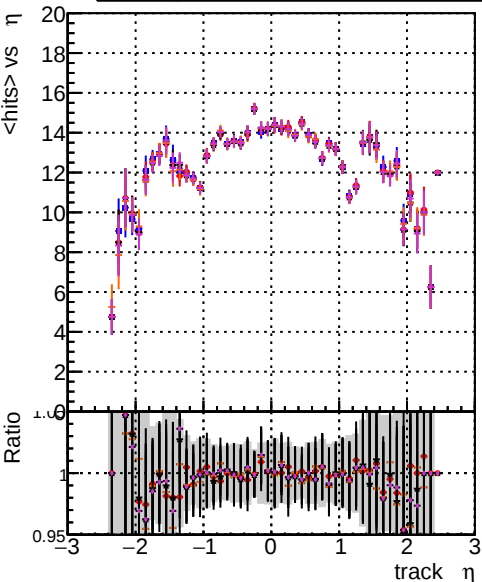
mean hits vs \eta DOM CKFEEIT 1000evt DOM CKFEREIT 1000evt DOM CKFEEIT 10000evt DOM TESTOLHIT 1000evt DOM TESTOLHIT 10000evt-50000t
