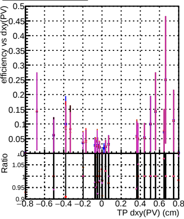
Efficiency vs Dxy(PV) DQM_CKFFit_1000evt DQM_CKFREFit_1000evt DQM_MkFitREFit_1000evt DQM_TESTOLHIT_1000evt DQM_TESTOLHIT_1000evt-50000t
