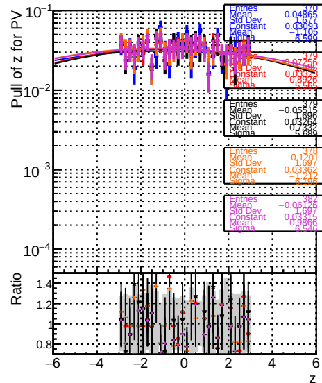
RecoPVAssoc2GenPVMatched_PullZ
