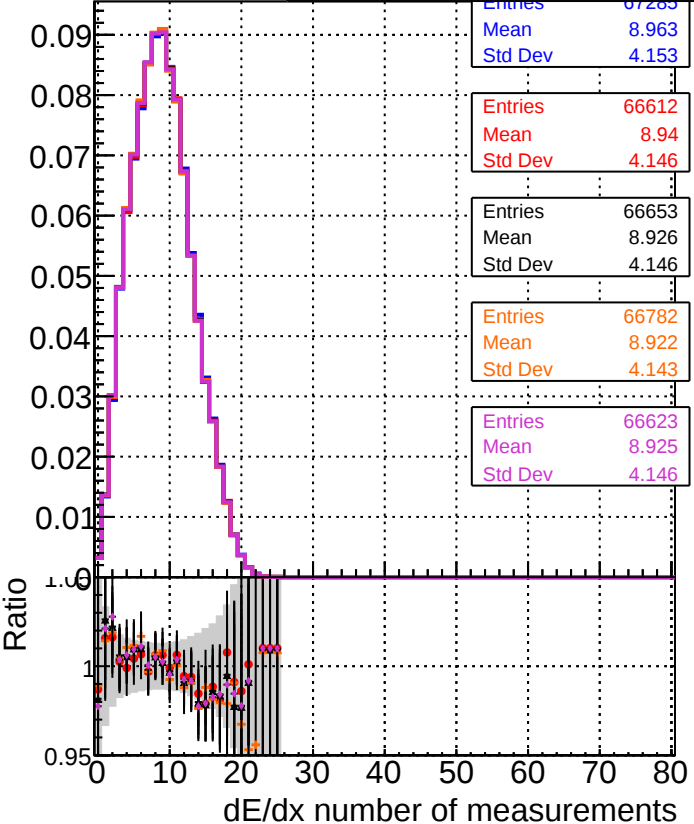
DOM_CKFFit_1000evt DOM_CKFREFit_1000evt DOM_MkFitREFit_1000evt DOM_TESTOLHIT_1000evt DOM_TESTOLHIT_1000evt-50000t
