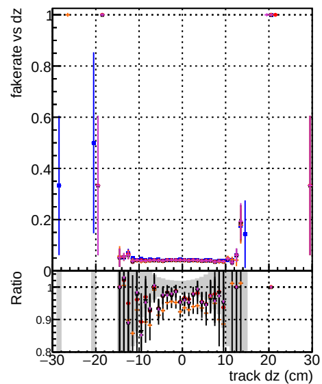
Fake rate vs dz DOM CKFit 1000evt DOM CKFit 5000evt DOM CKFit 10000evt DOM YES+OENIT 10000evt-50000t
