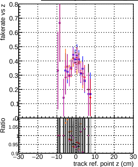
Fake rate vs v DOM CKFit 1000evt DOM CKFit 10000evt DOM CKFit 100000evt DOM CKFit 1000000evt TEST OHIT 10000evt
