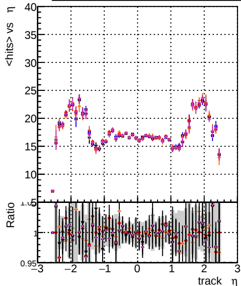
mean hits vs \eta DOM CKFEE1 1000evt DOM CKFEE1 10000evt DOM CKFEE1 100000evt DOM TESTOLHIT 1000evt DOM TESTOLHIT 10000evt DOM TESTOLHIT 100000evt
