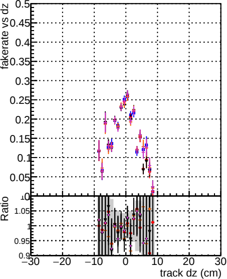
Fake rate vs dz DOM CKFit 1000evt DOM CKFit 5000evt DOM CKFit 10000evt DOM CKFit 50000evt
