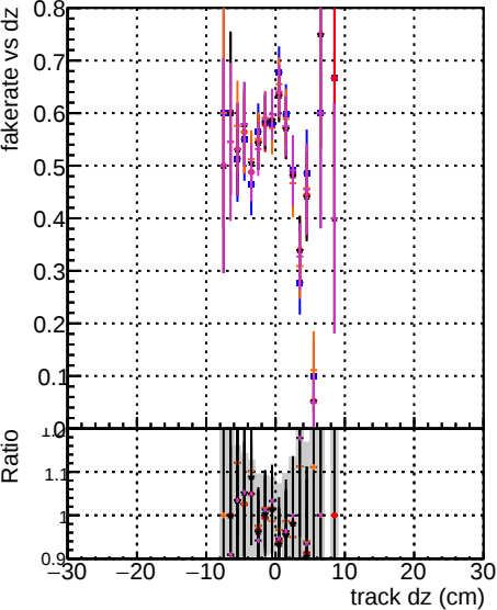
Fake rate vs dz DOM CKFit 1000evt DOM CKFit 5000evt DOM CKFit 10000evt DOM YES10Fit 10000evt DOM YES10Fit 50000evt
