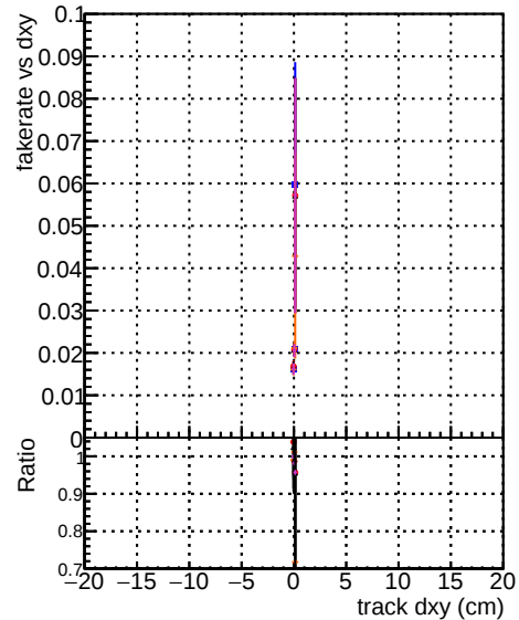
Fake rate vs d Legend: DGM CKF5it-1000evt DGM CKF5it-1000evt-50000 DGM CKF5it-1000evt-100000 DGM TEST0Hit-1000evt-50000
