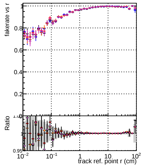
Fake rate vs DQM CKFEEFit 1000evt DQM CKFEEFit 1000evt DQM CKFEEFit 1000evt DQM TESTOLHIT 1000evt-50000t
