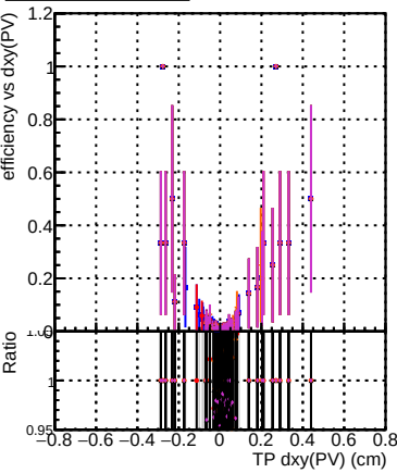
Efficiency vs Dxy(PV) DOM_CKFFit_1000evt DOM_CKFREFit_1000evt DOM_MkFitREFit_1000evt DOM_TESTOLHIT_1000evt DOM_TESTOLHIT_1000evt-50000t
