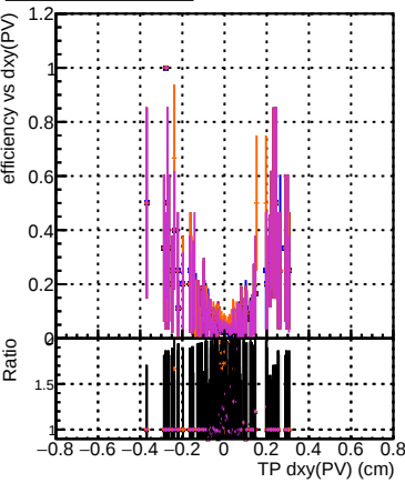
Efficiency vs Dxy(PV) Legend: DOM_CKFit_1000evt DOM_CKFREFit_1000evt DOM_MkFitREFit_1000evt DOM_TESTOLHIT_1000evt DOM_TESTOLHIT_1000evt-50000t
