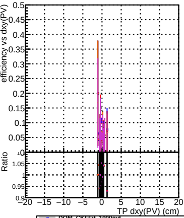
Efficiency vs Dxy(PV) (cm) Legend: DOM_CKFit_1000evt DOM_CKFREFit_1000evt DOM_MkFitREFit_1000evt DOM_TESTOLHIT_1000evt DOM_TESTOLHIT_1000evt-50000t
