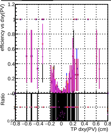
Efficiency vs Dxy(PV) (cm) Legend: DOM_CKFit_1000evt DOM_CKFREFit_1000evt DOM_MkFitREFit_1000evt DOM_TESTOLHIT_1000evt DOM_TESTOLHIT_1000evt-50000t
