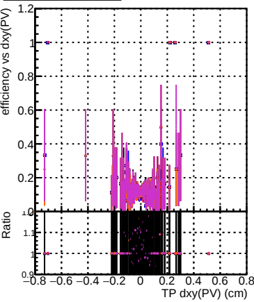
Efficiency vs Dxy(PV) Legend: DQM_CKFit_1000evt DQM_CKFREFit_1000evt DQM_MkFitREFit_1000evt DQM_TESTOLHIT_1000evt DQM_TESTOLHIT_1000evt-50000t
