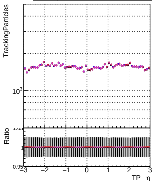
N of sin \leftarrow DOM-MkFitREFit 1000evt N of sin \leftarrow DOM-TESTOLHIT 1000evt N of sin \leftarrow DOM-TESTOLHIT 1000evt-1000t
