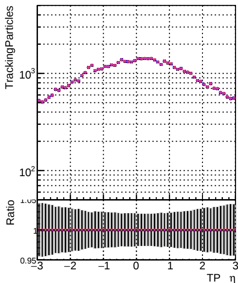
N of sin Legend DOM-MkFitREFit 1000evt DOM-TESTOLHIT 1000evt DOM-TESTOLHIT 1000evt-1000t
