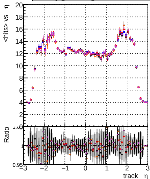
mean hits vs \eta DOM CKFFIT 1000evt DOM CKFFIT 10000evt DOM CKFFIT 100000evt DOM TESTOLHIT 1000evt DOM TESTOLHIT 10000evt DOM TESTOLHIT 100000evt
