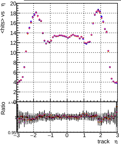
mean hit \eta DOM CKFEEL 1000evt DOM CKFEEL 1000evt DOM CKFEEL 1000evt DOM TESTOLHIT 1000evt DOM TESTOLHIT 1000evt-1000t
