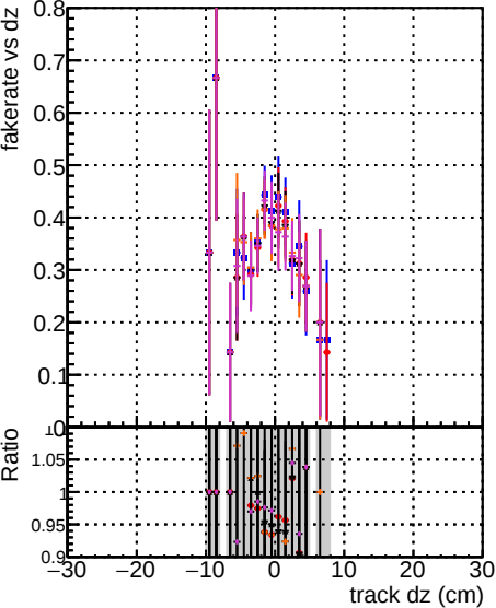
Fake rate vs dz DOM CKFit 1000evt DOM CKFit 5000evt DOM CKFit 10000evt DOM YES Fit 10000t
