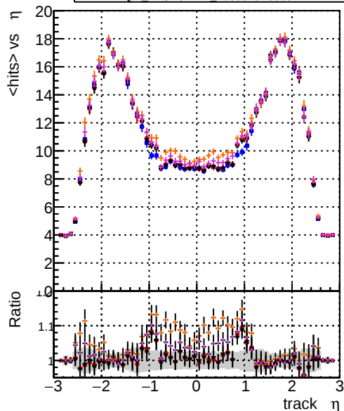
mean hits vs \eta DOM CKFit 1000evt DOM CKFit 10000evt DOM CKFit 100000evt DOM TESTOLHIT 1000evt DOM TESTOLHIT 10000evt DOM TESTOLHIT 100000evt
