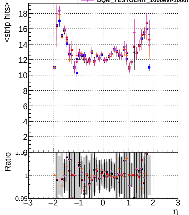
mean # STRIP hits vs eta
