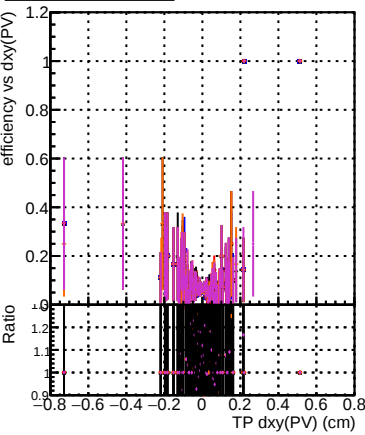
Efficiency vs Dxy(PV) (cm) Legend: DQM_CKFit_1000evt DQM_CKFREFit_1000evt DQM_MkFitREFit_1000evt DQM_TESTOLHIT_1000evt DQM_TESTOLHIT_1000evt-1000t
