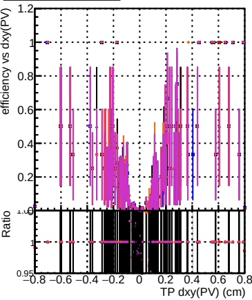
Efficiency vs Dxy(PV) (cm) Legend: DQM_CKFFit_1000evt DQM_CKFREFit_1000evt DQM_MkFitREFit_1000evt DQM_TESTOLHIT_1000evt DQM_TESTOLHIT_1000evt-1000t
