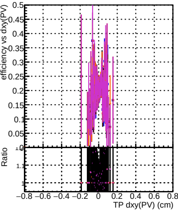
Efficiency vs Dxy(PV) (cm) DOM_CKFFit_1000evt DOM_CKFREFit_1000evt DOM_MkFitREFit_1000evt DOM_TESTOLHIT_1000evt DOM_TESTOLHIT_1000evt-1000t
