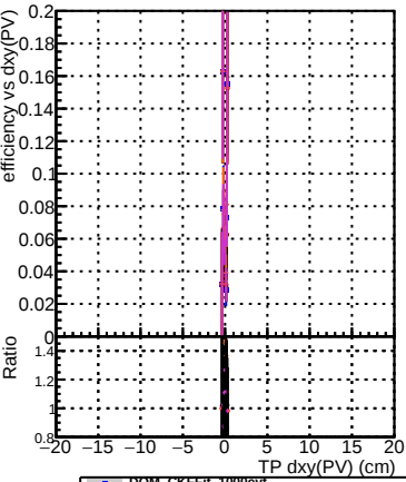
Efficiency vs Dxy(PV) Legend: DOM_CKFFit_1000evt DOM_CKFREFit_1000evt DOM_MkFitREFit_1000evt DOM_TESTOLHIT_1000evt DOM_TESTOLHIT_1000evt-1000t
