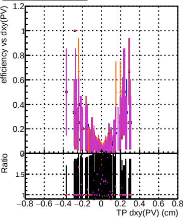
Efficiency vs Dxy(PV) Legend: DOM_CKFFit_1000evt DOM_CKFREFit_1000evt DOM_MkFitREFit_1000evt DOM_TESTOLHIT_1000evt DOM_TESTOLHIT_1000evt-1000t
