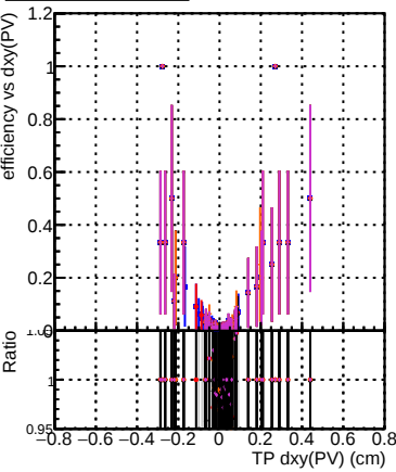
Efficiency vs Dxy(PV) Legend: DQM_CKFit_1000evt DQM_CKFREFit_1000evt DQM_MkFitREFit_1000evt DQM_TESTOLHIT_1000evt DQM_TESTOLHIT_1000evt-1000t
