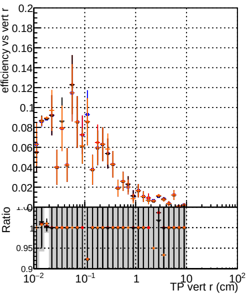
Efficiency vs TP vert r (cm) DOM_CKFFit_1000evt DOM_CKFREFit_1000evt DOM_MkFitREFit_1000evt DOM_TESTOLHIT_1000evt
