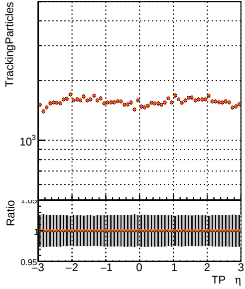
—●— DQM_CKFFit_1000evt —●— DQM_CKFREFit_1000evt —●— DQM_MkFitREFit_1000evt —●— DQM_TESTOLHIT_1000evt
