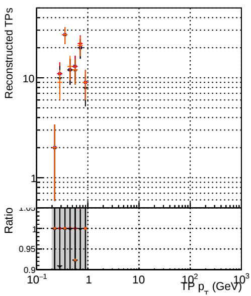
—●— DQM_CKFFit_1000evt —●— DQM_CKFREFit_1000evt —●— DQM_MkFitREFit_1000evt —●— DQM_TESTOLHIT_1000evt
