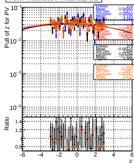
RecoPVAssoc2GenPVMatched_PulIZ
