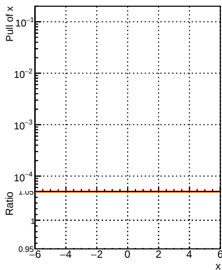
RecoAllAssoc2GenMatched_PulIX
