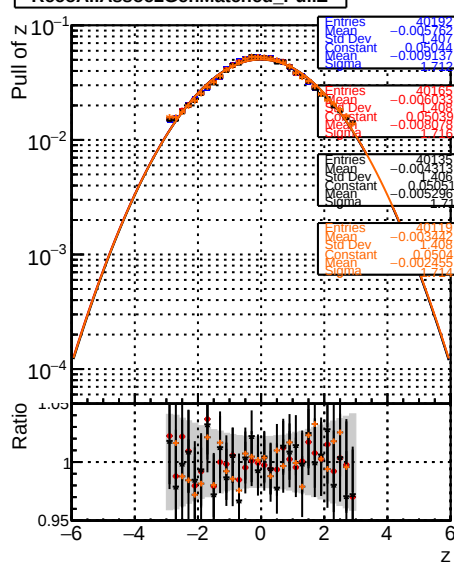
RecoAllAssoc2GenMatched_PulIZ
