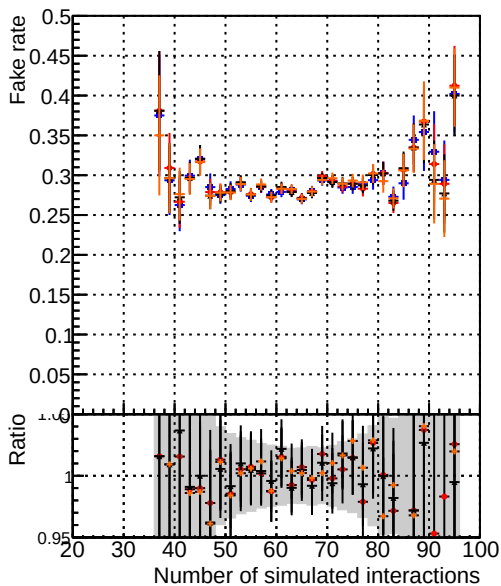
Fakerrate vs PU
