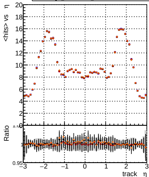
mean hits vs \eta DOM_CKFFit_1000evt DOM_CKFFit_1000evt DOM_MkFitREFit_1000evt DOM_TESTOLHIT_1000evt
