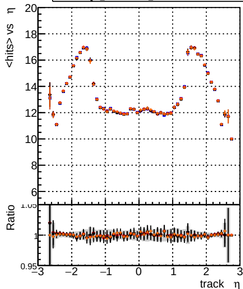
mean hits DOM_CKFFit_1000evt DOM_CKFREFit_1000evt DOM_MkFitREFit_1000evt DOM_TESTOLHIT_1000evt
