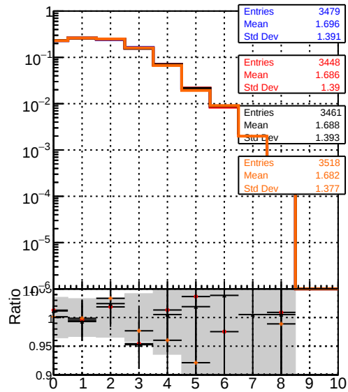
mean hits vs \eta DOM_CKFFit_1000evt DOM_CKFFit_1000evt DOM_MkFitREFit_1000evt DOM_TESTOLHIT_1000evt
