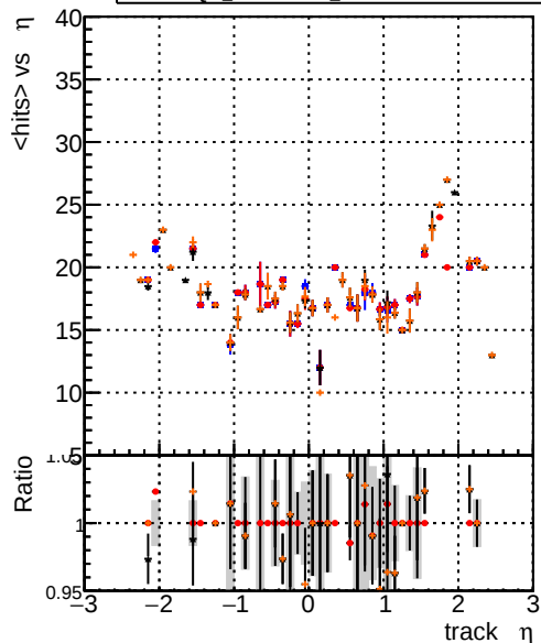
mean hit DOM_CKFFit_1000evt DOM_CKFREFit_1000evt DOM_MkFitREFit_1000evt DOM_TESTOLHIT_1000evt
