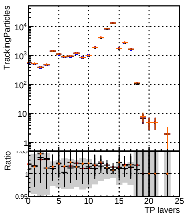
—●— DQM_MkFitREFit_1000evt —●— DQM_TESTOLHIT_1000evt
