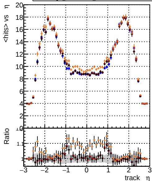
mean hits vs \eta DOM_CKFFit_1000evt DOM_CKFREFit_1000evt DOM_MkFitREFit_1000evt DOM_TESTOLHIT_1000evt
