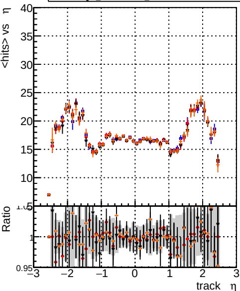
mean hit DOM_CKFFit_1000evt DOM_CKFREFit_1000evt DOM_MkFitREFit_1000evt DOM_TESTOLHIT_1000evt
