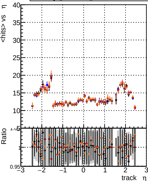
mean hits vs \eta DOM_CKFFit_1000evt DOM_CKFFit_1000evt DOM_MkFitREFit_1000evt DOM_TESTOLHIT_1000evt
