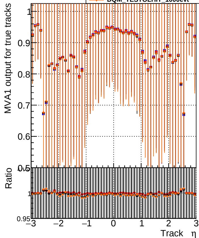
—■— DQM_CKFFit_1000evt —●— DQM_CKFREFit_1000evt —▲— DQM_MkFitREFit_1000evt —◆— DQM_TESTOLHIT_1000evt
