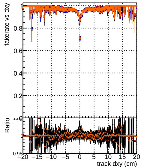
Fake rate vs d BSM CKEFit 1000evt BSM CKEFit 1000evt BSM TEST0EHT 1000evt
