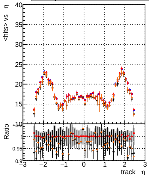
mean hit DOM_CKFFit_1000evt DOM_CKFREFit_1000evt DOM_MkFitREFit_1000evt DOM_TESTOLHIT_1000evt
